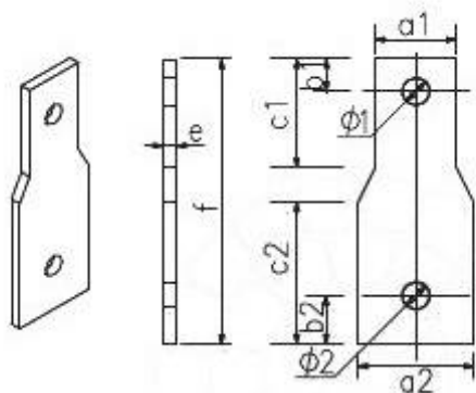
A/C相用转接铜排
