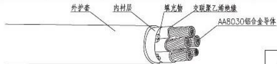
ZC-TC90(-40)示意图
