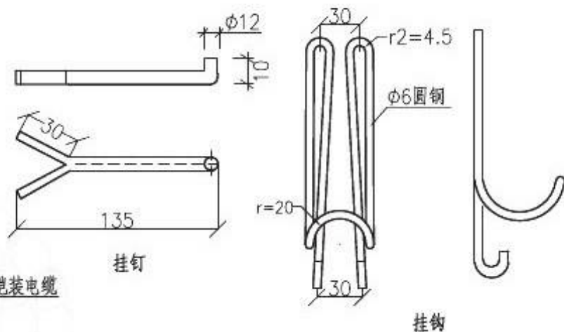
电缆沿墙面敷设方式II
