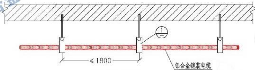
单根电缆沿吊架敷设
