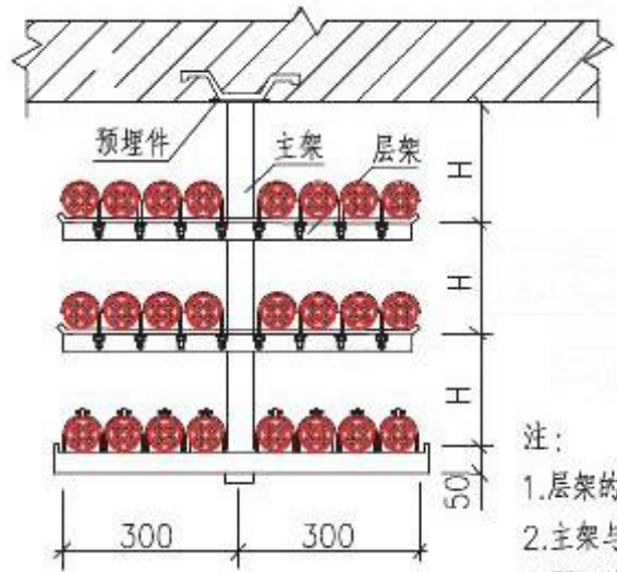
楼板下吊架敷设
