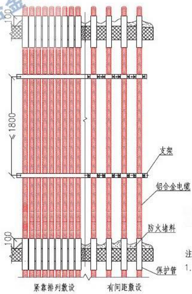
铝合金铠装电缆垂直敷设
