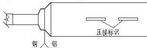
针形铜铝过渡端子
