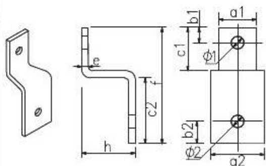
B相用转接铜排
