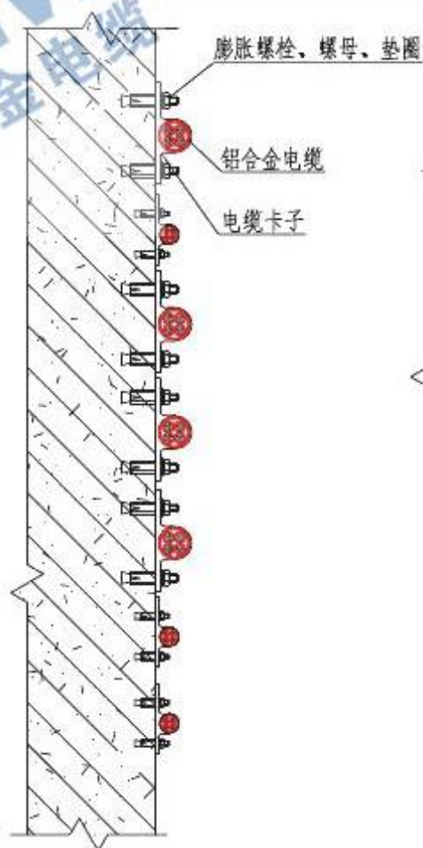
电缆沿墙面敷设方式I
