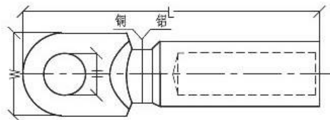
CAU型铜铝过渡端子
