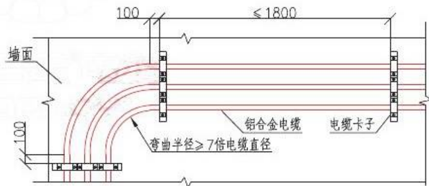
电缆沿墙面敷设方式II
