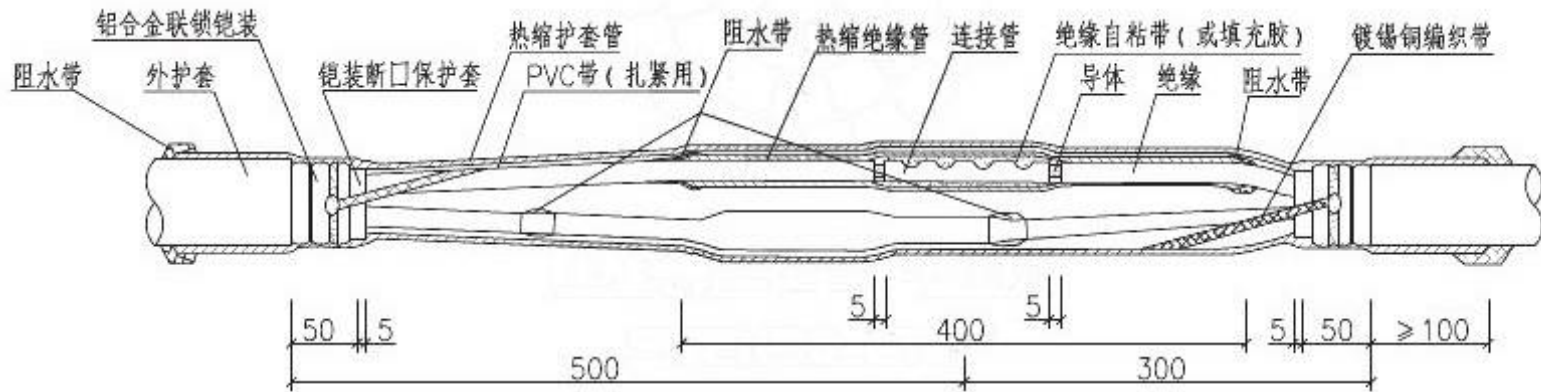
热缩型电缆接头
