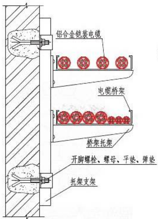
沿梯架水平敷设
