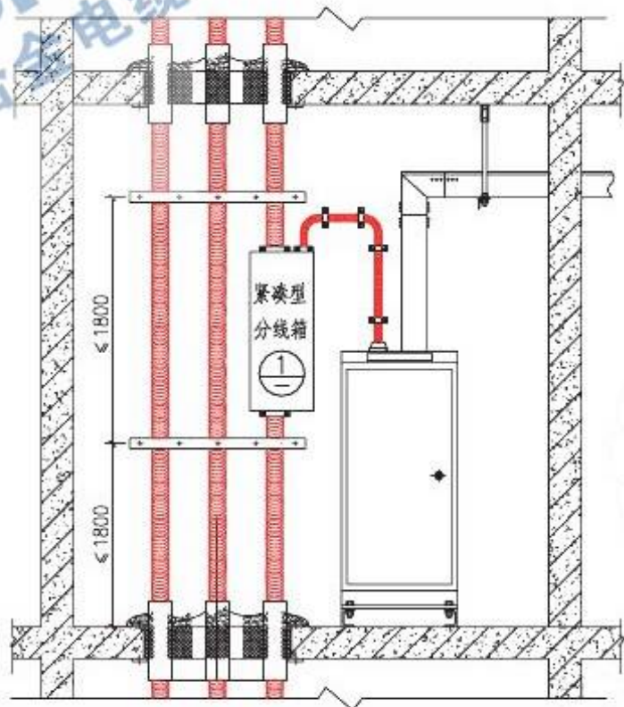
紧凑型分线箱内部安装图
