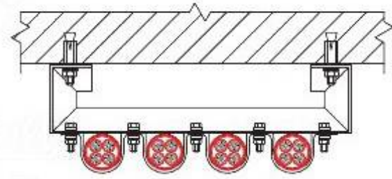
单层电缆沿吊架敷设
